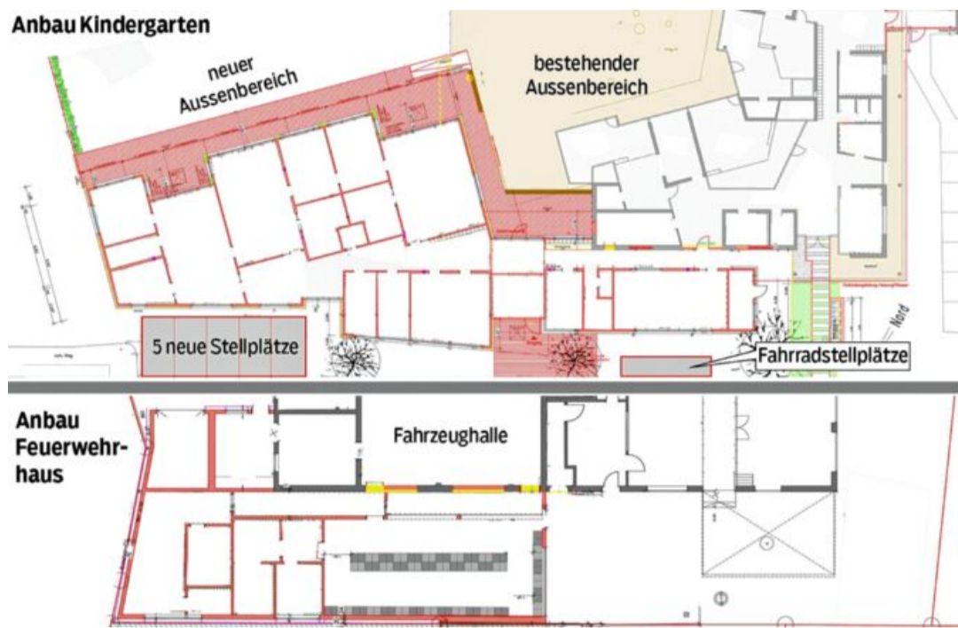
Die Planskizzen: Oben der Anbau an den Kindergarten in Verlängerung der Albstraße. Unten die Erweiterung des Feuerwehrhauses in Richtung Nordwesten. Gestaltung: ca
